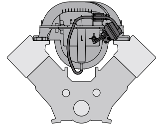
Múltiple de admisión con tubos variables en un motor en V
