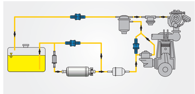
应用示例：带有切换式电动附加泵的化油器发动机
