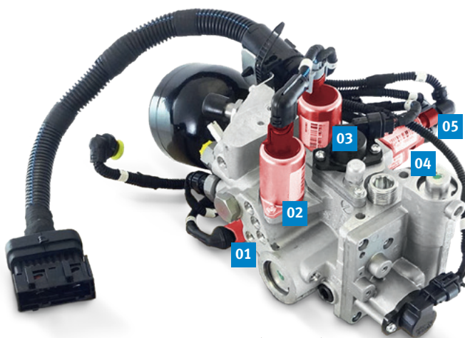
01-05 Cinq clapets de commande (en rouge) sur une boîte de vitesses Selespeed
