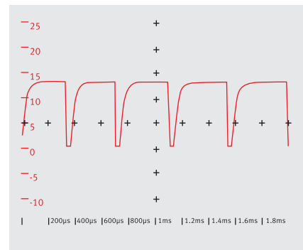
Señal en régimen de ralentí (en función de la velocidad de la marcha en ralentí)
