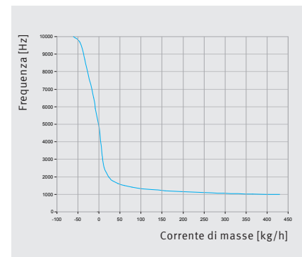
Diagramma caratteristico sensore corrente
