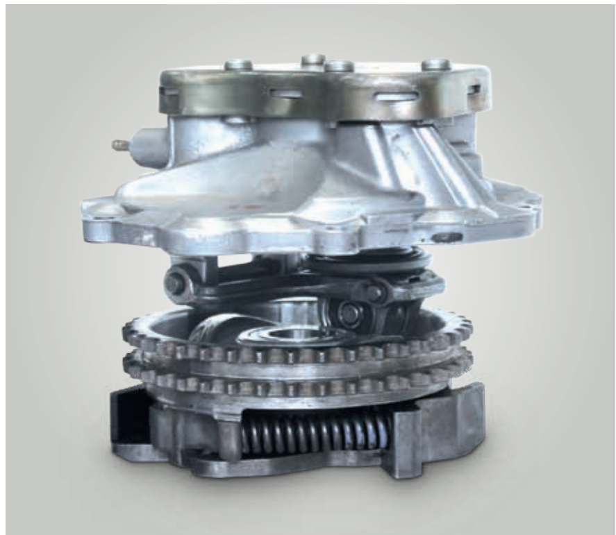
Вакуумные насосы серии 7.20607 ... (сверху) на муфте опережения впрыскивания
