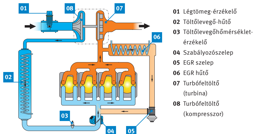
2. ábra: A hűtött füstgáz-visszavezetés sémája
