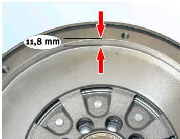
איור 2: 415 0239 10 \ 415 0243 10 (גרסא חדשה של גלגל תנופה כפול מסה)
