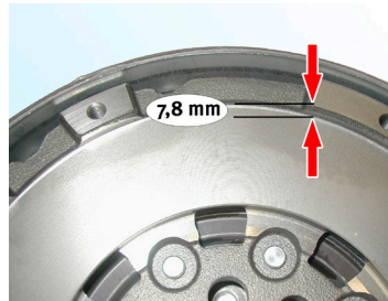
איור 1: 415 0148 10 \ 415 0151 10 (גרסא ישנה של גלגל תנופה כפול מסה)
