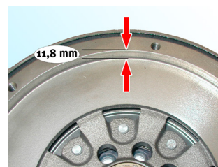
Bild 2: 415 0239 10 (nyare version av dubbelmassesvängghjul)
