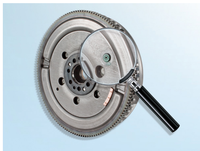
Figur 1: Transportsikringen forblir i tomassesvinghjulet
