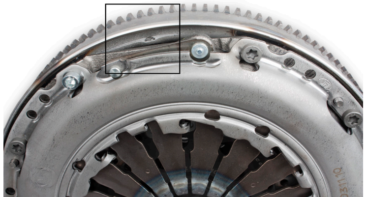
Slika 1: Tragovi utisnuća predugog vijka na površini materijala primarne mase
