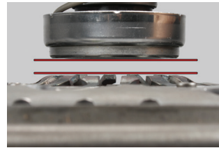
Resim 3: Doğru montaj
