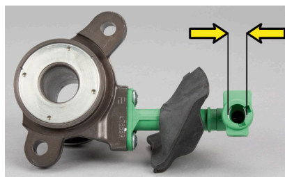
Obrázek 4: LuK CSC 510 0137 10 Hydraulická přípojka 12,2 mm
