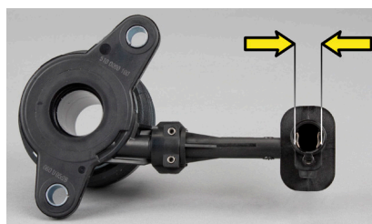
Obrázek 1: LuK CSC 510 0090 10 Hydraulická přípojka 12,2 mm
