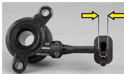
Obrázek 2: LuK CSC 510 0097 10 Hydraulická přípojka 13,3 mm
