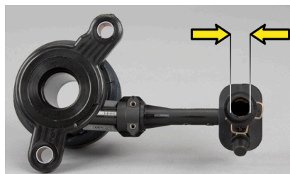
Billede 3: LuK CSC 510 0098 10 Hydraulisk tilslutning 11,7 mm
