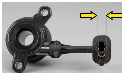
Billede 2: LuK CSC 510 0097 10 Hydraulisk tilslutning 13,3 mm
