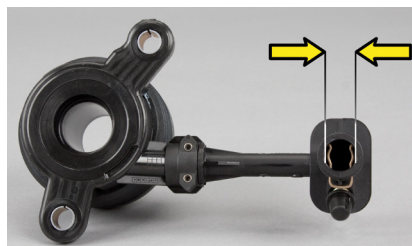
Figur 2: LuK CSC 510 0097 10 hydraulisk tilkobling 13.3 mm
