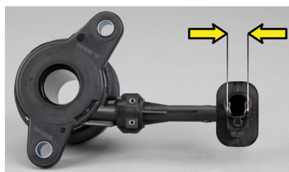
Figur 1: LuK CSC 510 0090 10 hydraulisk tilkobling 12.2 mm
