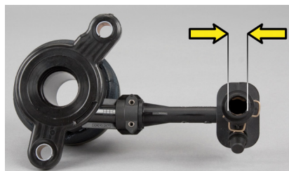
Figur 3: LuK CSC 510 0098 10 hydraulisk tilkobling 11.7 mm
