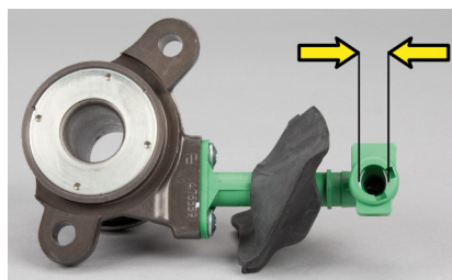
Figur 4: LuK CSC 510 0137 10 hydraulisk tilkobling 12.2 mm
