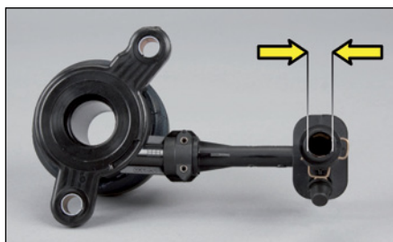
Foto 3: Centralny wysprzęglik LuK 510 0097 10 przyłączy hydrauliczne 13.3 mm
