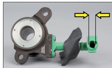
Foto 4: Centralny wysprzęglik LuK 510 0137 10 przyłączy hydrauliczne 12.2 mm
