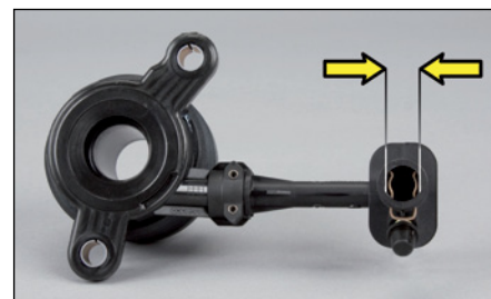
Foto 2: Centralny wysprzęglik LuK 510 0098 10 przyłączy hydrauliczne 11.7 mm
