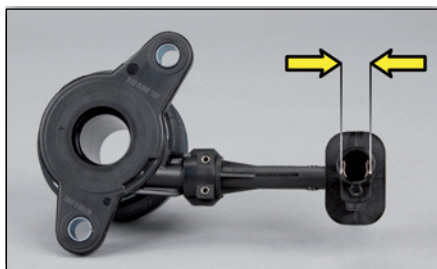
Foto 1: Centralny wysprzęglik LuK 510 0090 10 przyłączy hydrauliczne 12.2 mm
