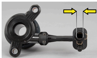
Fig. 3: Conexiune hidrolică LuK CSC 510 0098 10 de 11,7 mm
