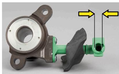
Fig. 4: Conexiune hidrolică LuK CSC 510 0137 10 de 12,2 mm
