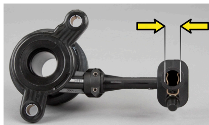
Fig. 2: Conexiune hidrolică LuK CSC 510 0097 10 de 13,3 mm
