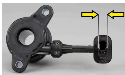
Fig. 1: Conexiune hidrolică LuK CSC 510 0090 10 de 12,2 mm
