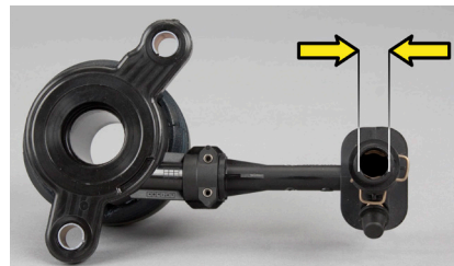
Зображення 3: Гідравлічний витискний підшипник LuK 510 0098 10 з гідравлічною муфтою 11,7 мм
