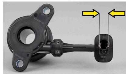
Зображення 1: Гідравлічний витискний підшипник LuK 510 0090 10 з гідравлічною муфтою 12,2 мм
