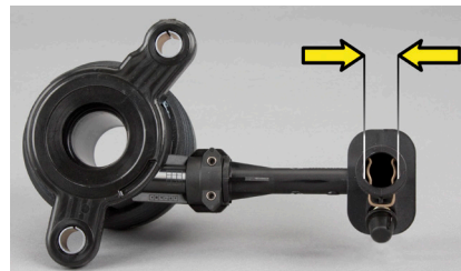
Зображення 2: Гідравлічний витискний підшипник LuK 510 0097 10 з гідравлічною муфтою 13,3 мм
