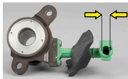
Зображення 4: Гідравлічний витискний підшипник LuK 510 0137 10 з гідравлічною муфтою 12,2 мм
