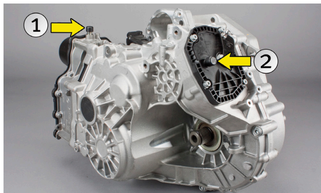
1. ábra: Közvetlen kapcsolású sebességváltó szellőzőkupakkal a mechatronika (1) és a sebességváltó (2) számára
