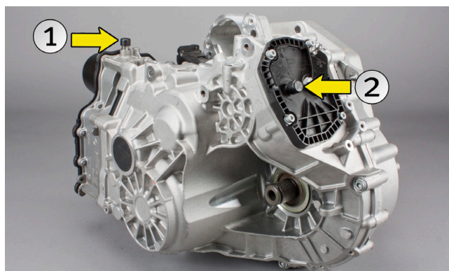
Рисунок 1: Преселективная коробка передач - вентиляционные колпачки на блоке мехатроники (1) и КПП (2)
