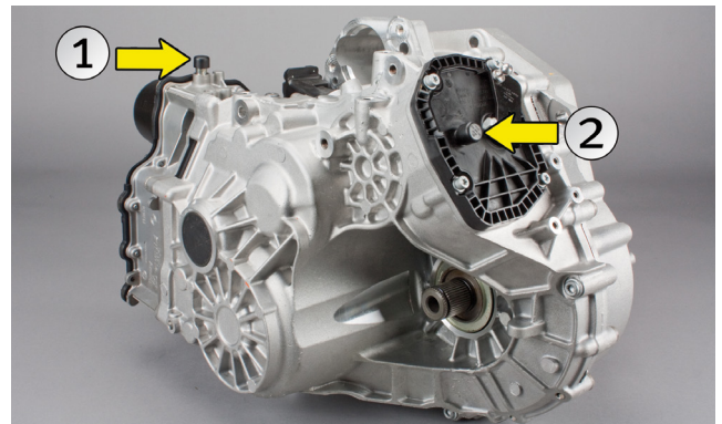
Bild 1: Direktväxlande växellåda med avluftningslock för mekatronikenhet (1) och växellåda (2)
