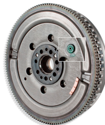
Рисунок 1: Двухмассовый маховик LuK со стопорным штифтом в качестве транспортного зажима
