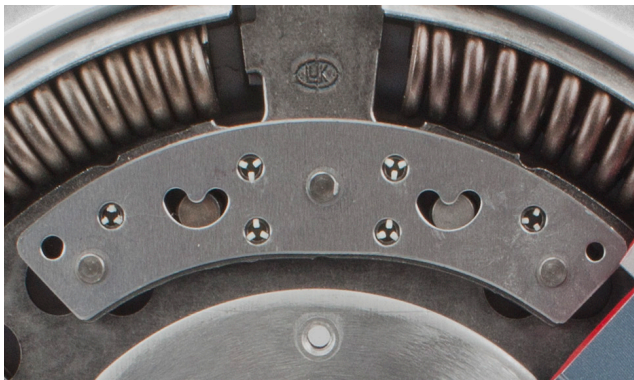
Billede 2: Centrifugalkraftpendul
