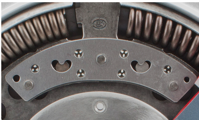
Εικόνα 2: Εκκρεμές φυγοκεντρικής δύναμης
