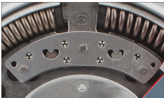
Fig. 2: Beweegbare centrifugaalpendel
