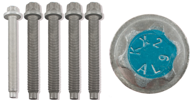
Figur 1: Kjøretøyproduzentens aluminiumskruesett (OE-nr.: 23 00 0 392 607)
