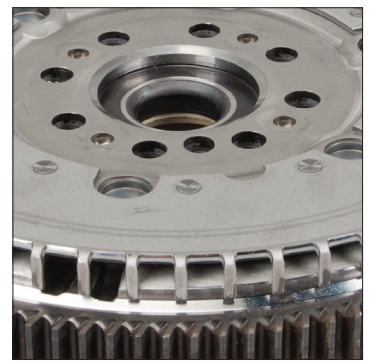
Fig. 2: Nieuwe uitvoering impulsring
