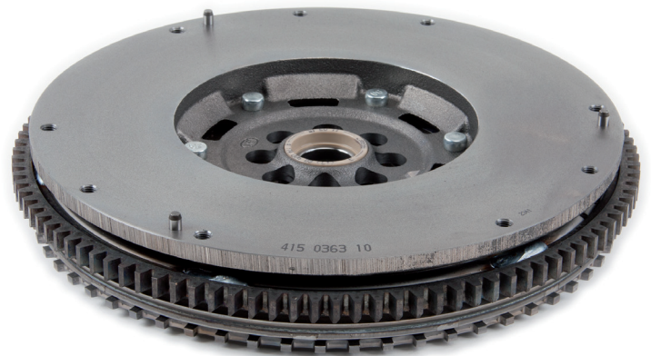
Fig. 1: Volante motor bimasa 415 0363 11 de LuK
