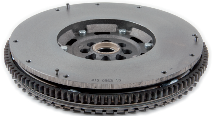
Volant bimasse de LuK réf. : 415 0363 11
