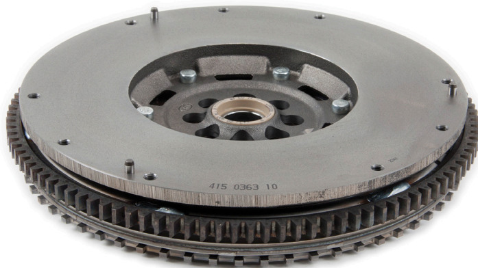
איור 1: גלגל תנופה כפול מסה מק"ט - 11 0363 415
