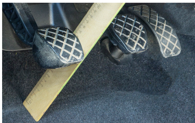
Fig. 1: După ce ambreiajul a fost înlocuit, se reglează jocul la pedală.
