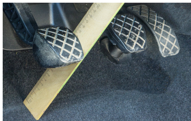
Bild 1: Efter kopplingsbyte skall pedalspelet ställas in.
