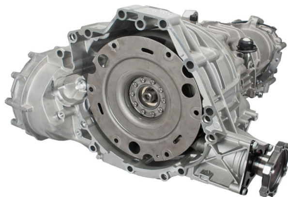
Fig. 1: Cutia de viteze cu modulul ambreiaj montat
