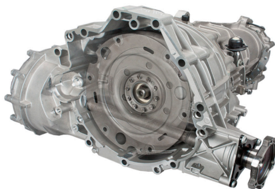
Obrázek 1: Spojovací hřídel přední nápravy probíhá mezi přenosovým plechem a dvouhmotovým setrvačником
