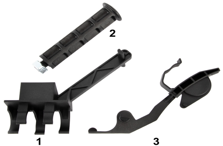
Fig. 2: Juego de herramientas de montaje con el número de artículo 400 0537 10
