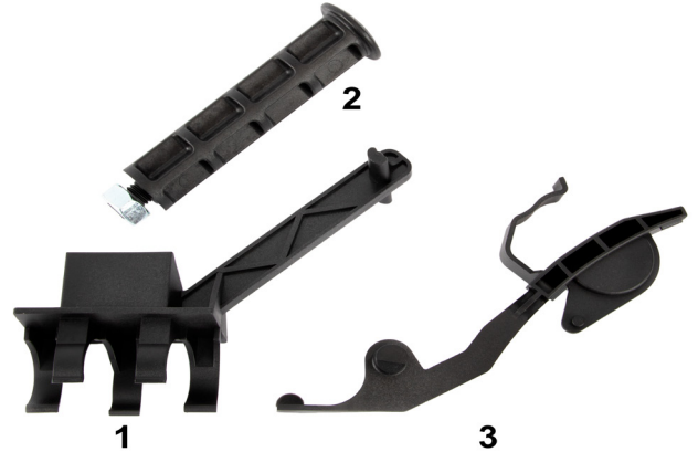
Kuva 2: Asennustyökalusarja tilausnumerolla 400 0537 10
