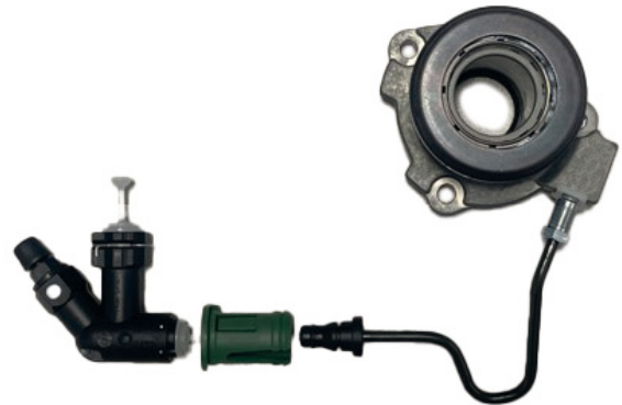
Imagen 2: Conducto hidráulico, piezas guía y piezas de conexión del fabricante del vehículo
