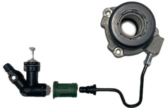
Afbeelding 2: Hydrauliekleiding, geleidings- en verbindingsonderdelen van de voertuigfabrikant
