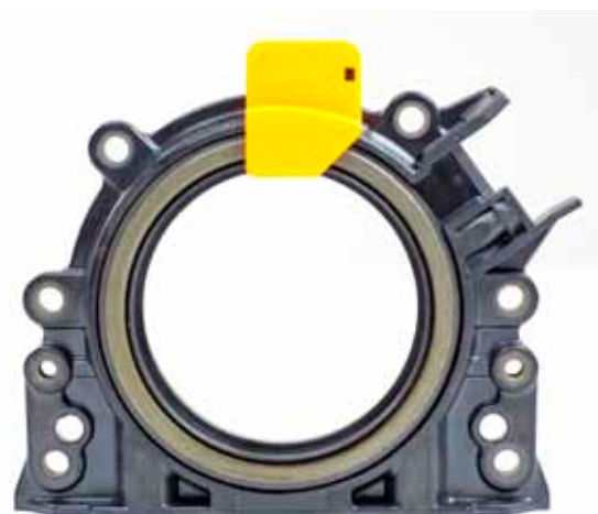
Fig. 2_Guarnizione ad anello incorporata
