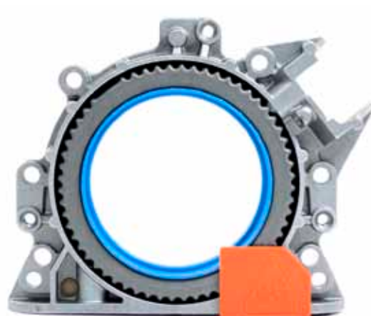
Fig. 1_Guarnizione ad anello incorporata
