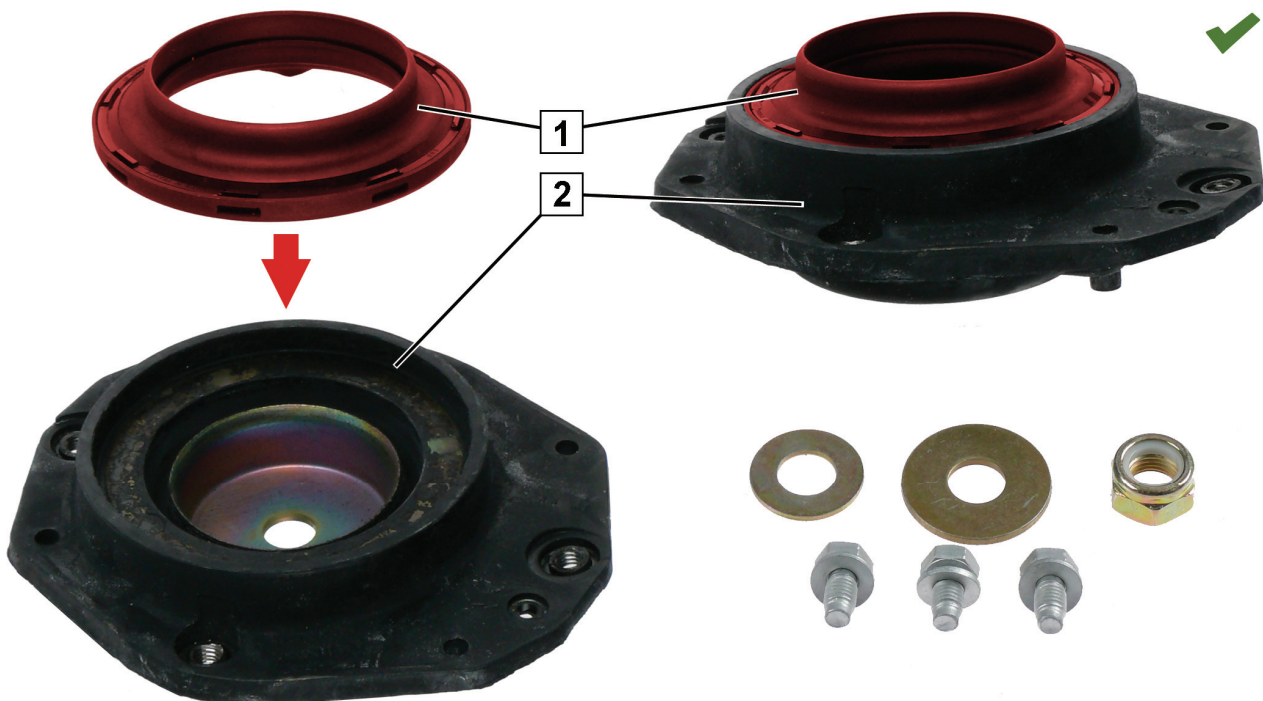
Fig. 3: Supporto superiore dell'ammortizzatore – montaggio corretto di cuscinetto volvente e componente in gomma-metallo
