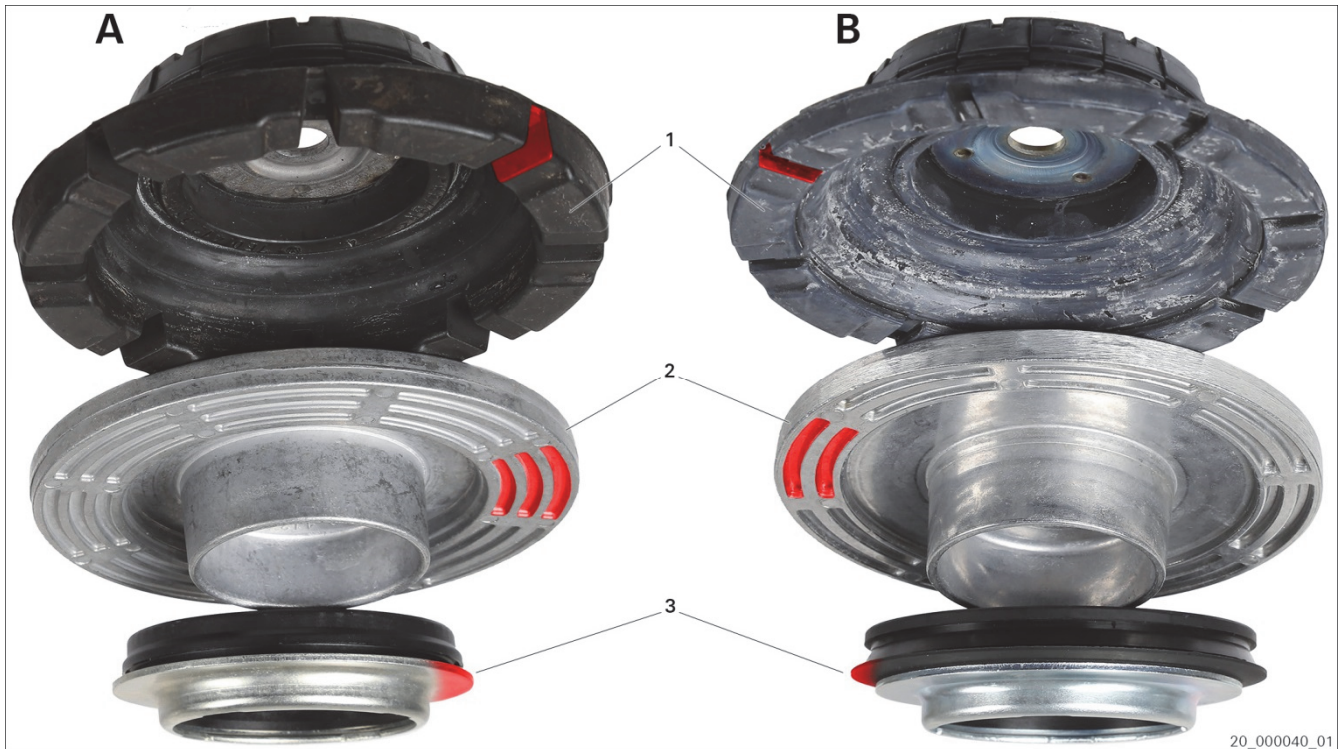
Obr. 1: Opěrné ložisko pružící jednotky variantu A/B
