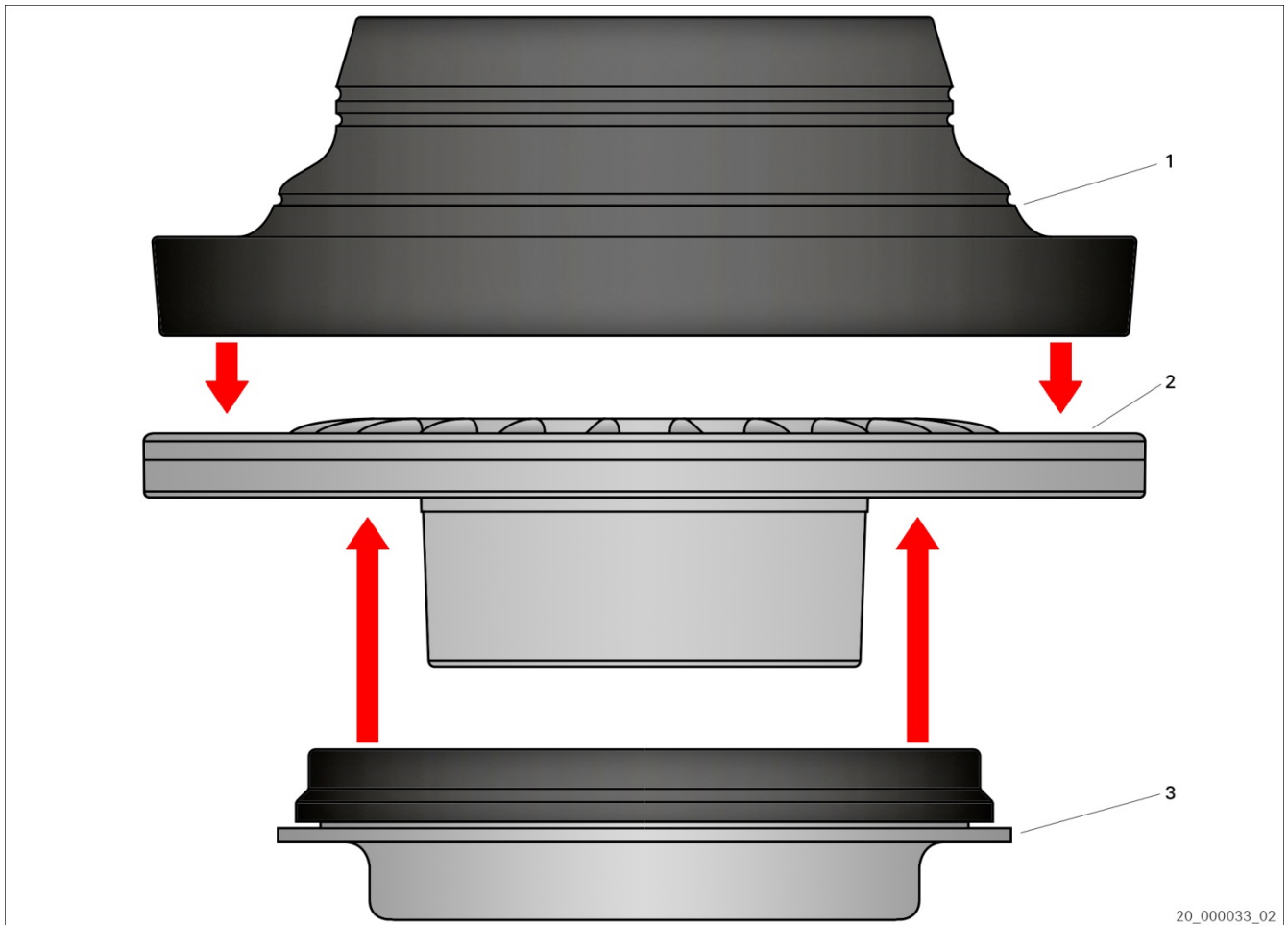
Εικ. 1: Συναρμολόγηση γονάτου ανάρτησης (παράδειγμα)
