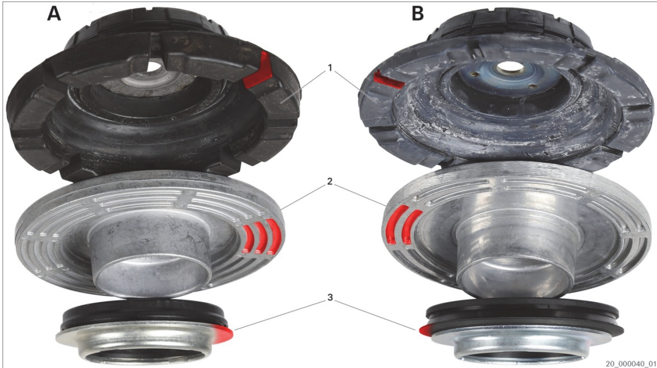
Εικ. 1: Έδρανο γόνατου ανάρτησης, τύπος A/B
