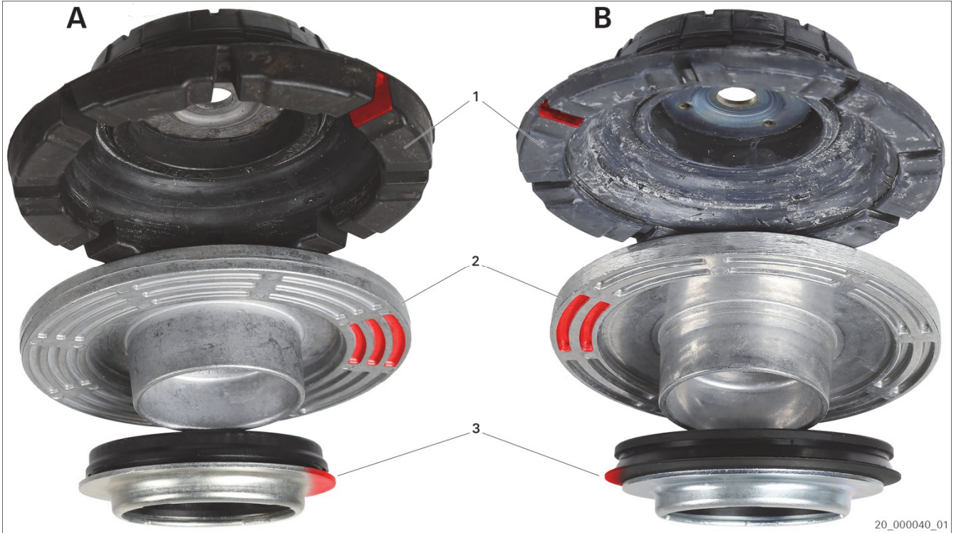
Şekil 1: Amortisör kule takozu Varyant A/B
