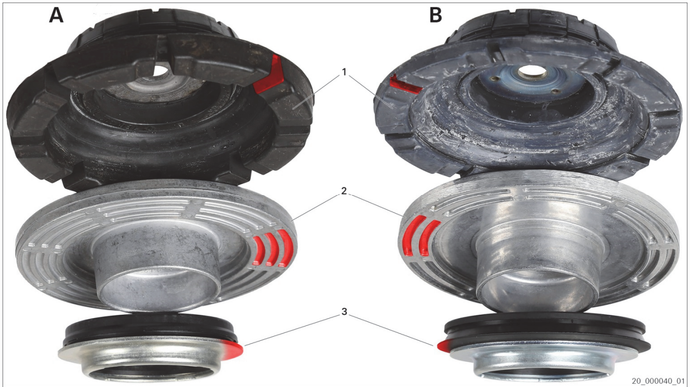
图示1：减振支柱座型号 A/B
