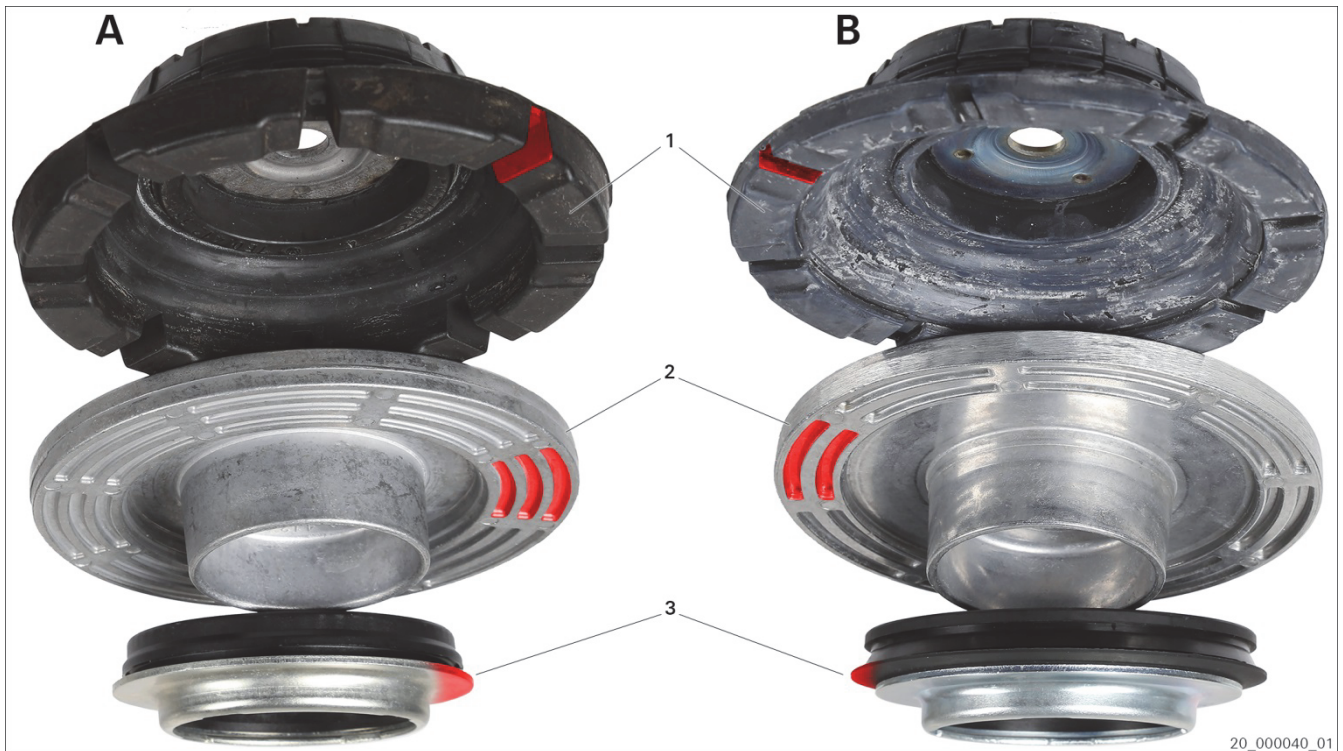
Фиг. 1: Опорен лагер на стойката на амортисьора варианти А/В
