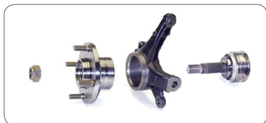
Ступичный узел HBU 2.1 и составные детали
