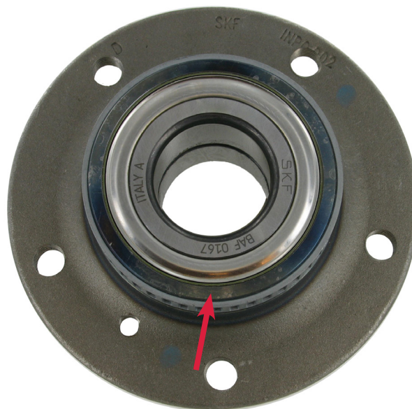
SKF design – kovové těsnění
