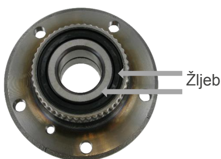
Aftermarket konstrukcija sa mono-zaptivkom i žljeb za štitnik od prašine
