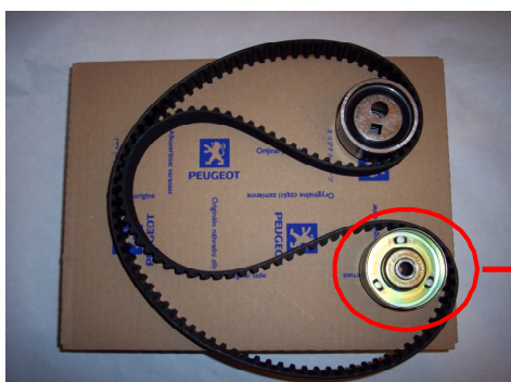
Contenu de l'ancien kit d'origine pour VKMA 03244/03247
