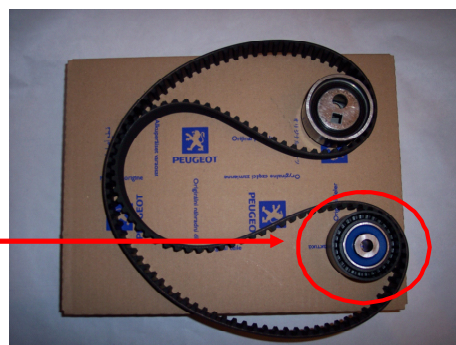
Contenu du nouveau kit d'origine pour VKMA 03244/03247
